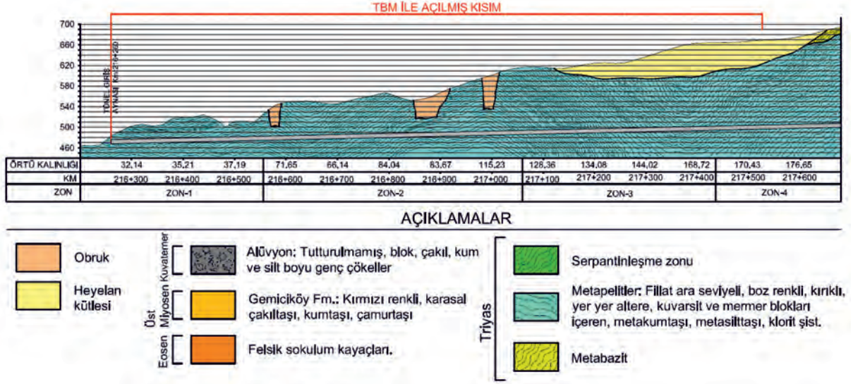
Şekil 9. Tünelin TBM ile açılan bölge ve bölümleri.
