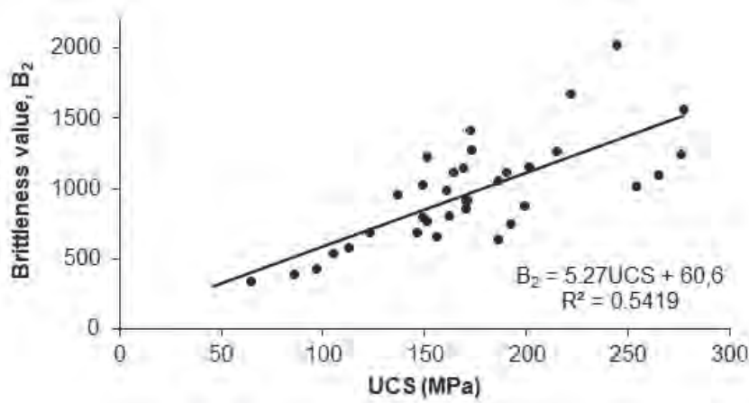
Şekil 7. Kayaçların gevreklik değeri ( B_2 ) ile tek eksenli sıkışma dayanımı arasındaki ilişki. Çizgisel olmayan ilişki kullanıldığında korelasyon katsayısı ( R^2 ) 0.68 olmaktadır.
