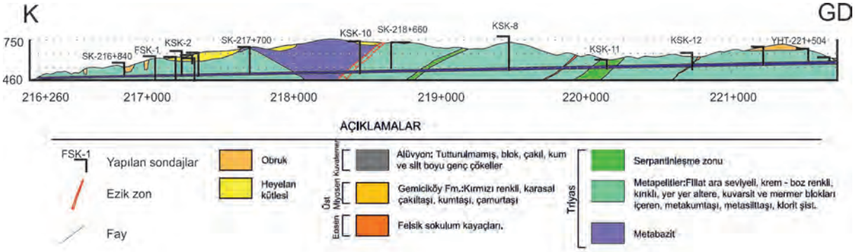
Şekil 7. İncelenen 26 numaralı tünelin boy kesiti (Tüysüz ve Genç, 2012'den değiştirilerek) (Tünel güzergahı kuzeyden başlayarak geniş bir karp ile K-G-GB-GD yönlerini kat etmektedir).
